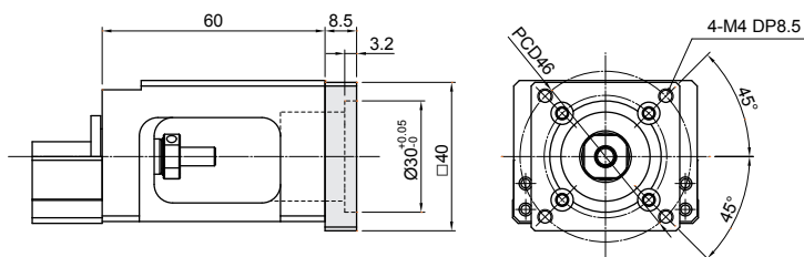
馬達連接法藍 F02
