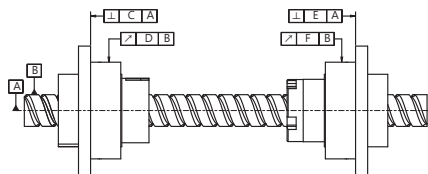
RFSY回転式ナット
