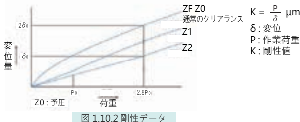
図 1.10.2 剛性データ
