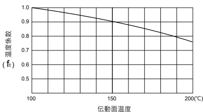
図 1.3.3 温度係数 (f t )
