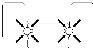
図 3.1.3 ゴシック 45° 4 方向荷重構造
