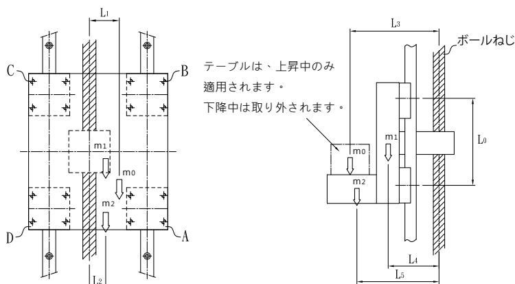
図 1.8.4 動作条件
