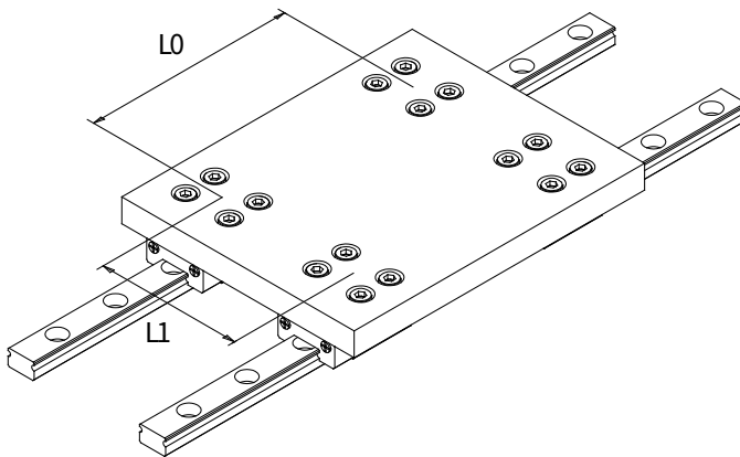
Fig 4.1.1 Span Dimensions
