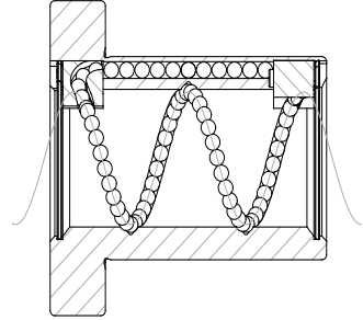
図 1.6.5 B タイプナット
