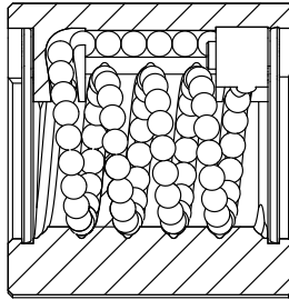
図 1.6.6 SQ 角形ボールねじナット
