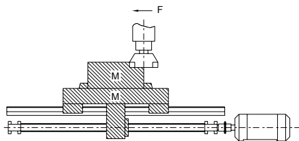
圖 1.5.1 負荷慣性矩
