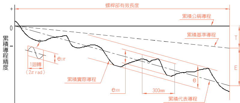
圖 1.3.1 導程精度之說明書 (ISO 3408)
