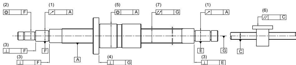
圖 1.3.2 滾珠螺桿安裝部位的精度 (ISO 3408)
