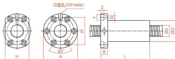
OFI 精密研磨級系列規格尺寸表
