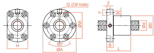
SFM 精密研磨級系列規格尺寸表
