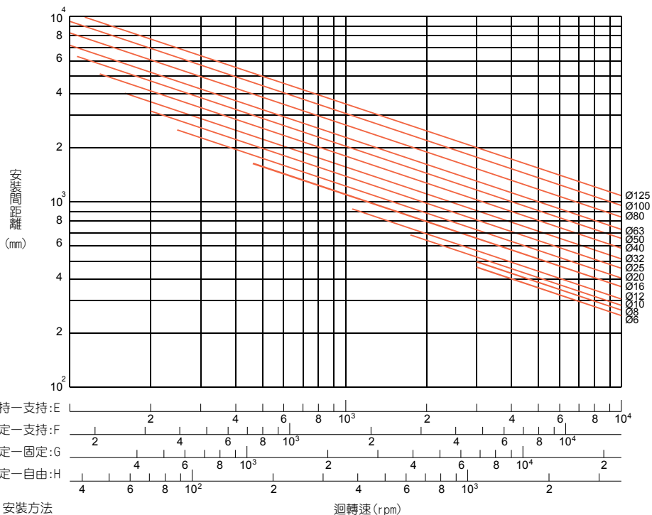
圖 1.4.17 軸對於危險速度之容許迴轉數
