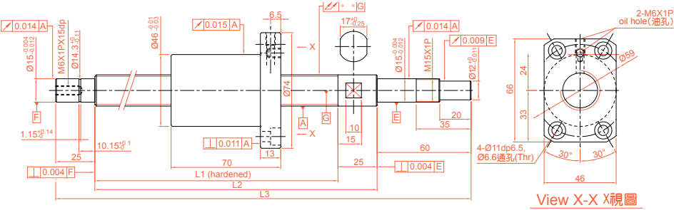
XSVR02020-00 精密研磨級系列規格尺寸表 ( 研磨級軸端完成品 )
