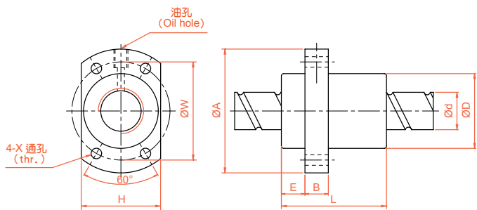
SFYA 轉造級系列規格尺寸表
