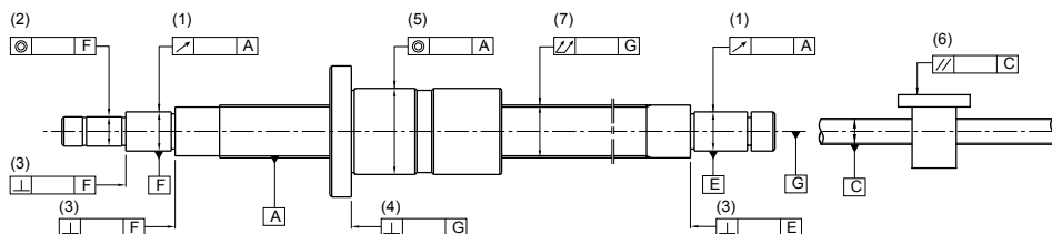
図 1.3.2 ボールねじの取り付け精度
