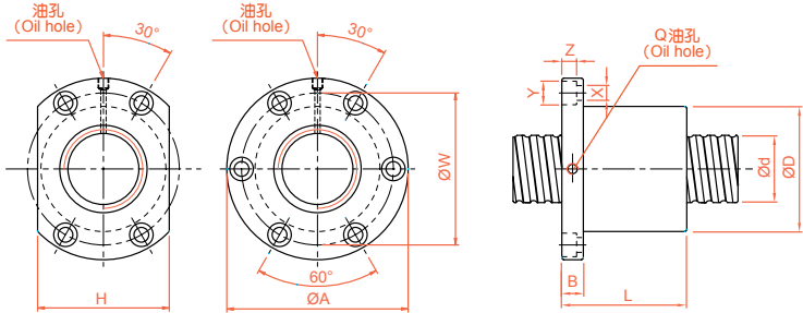
SFV 精密研磨級系列規格尺寸表
