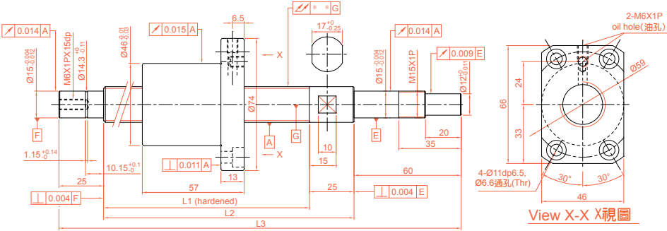
XSVR02010-00 精密研磨級系列規格尺寸表 ( 研磨級軸端完成品 )
