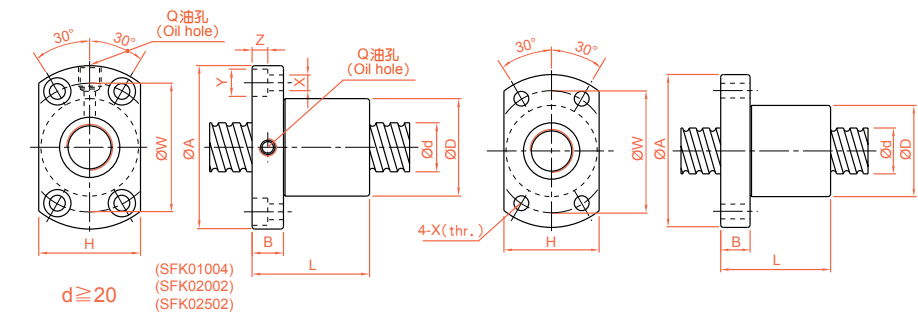
SFK 精密研磨級系列規格尺寸表
