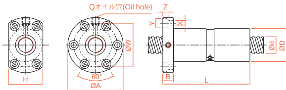
DFM 精密研削シリーズのサイズ規格
