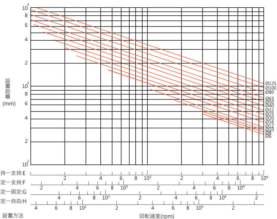
図 1.4.17 許容回転数線図
