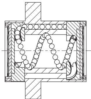
図 1.6.4 Y, H, A タイプナット
