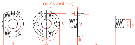
OFI/DFI 精密研削シリーズのサイズ規格
